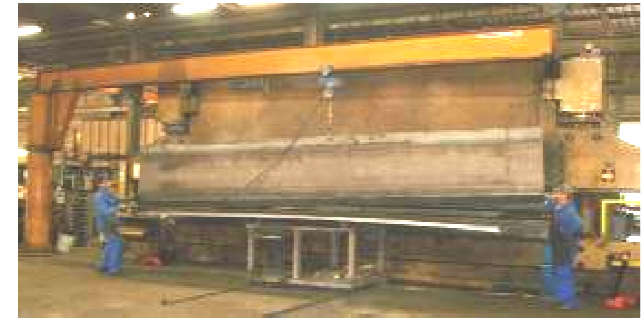
Presse plieuse 900 tonnes, Lg 7 mètres
